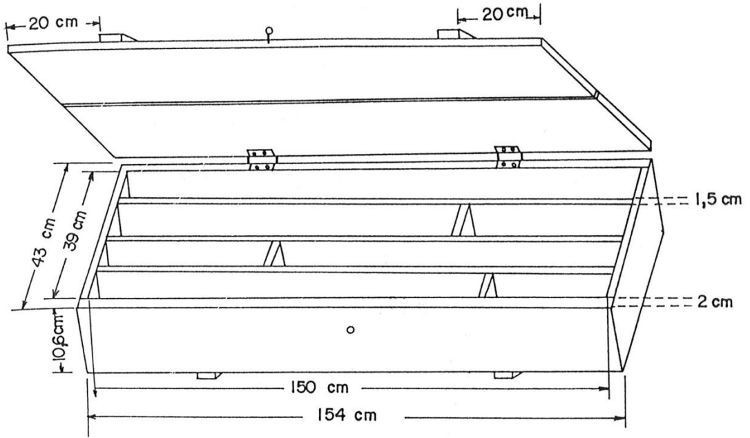
Şekil 1: Karot Sandığı Boyutları.
